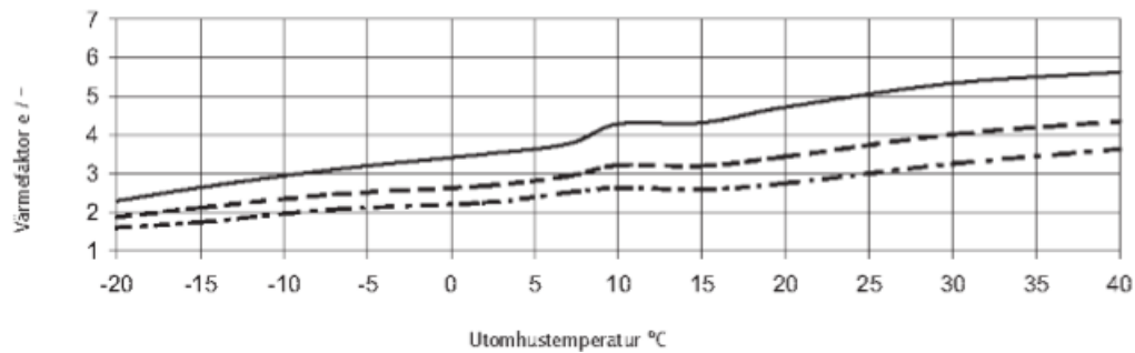
Figur 18: COP som funktion av utomhustemperatur. Figuren beskriver COP för WPL 23 som funktion av utomhustemperatur.
