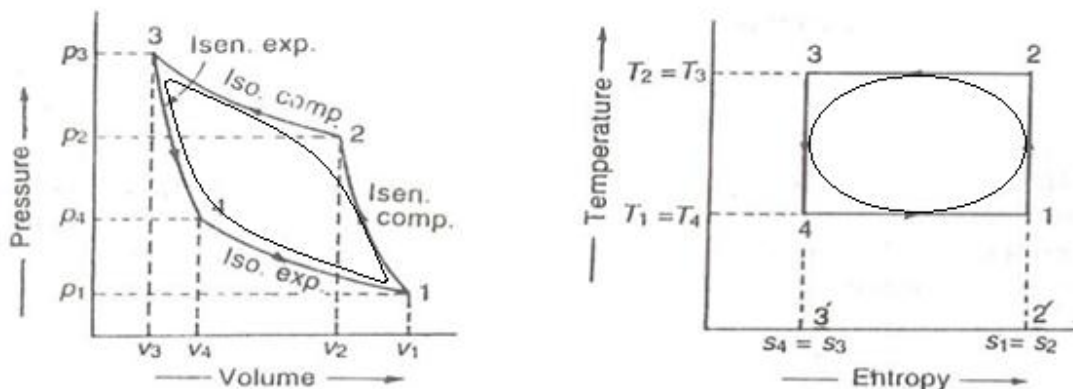
Figur 11: Pv- och ts-diagram för verklig kylmaskin/värmepumpprocess.
