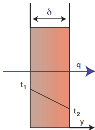
Figur 6: Värmeledning
