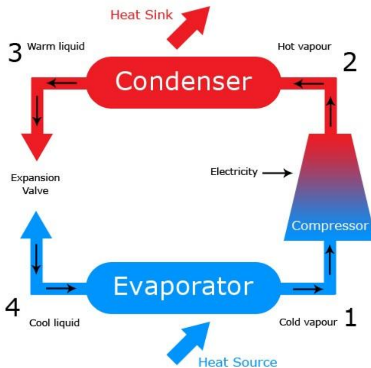
Figur 12: Förenklad processbild av ett värmepumpsystem 34
