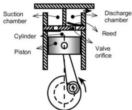
Figur 15: Kolvkompressor. 37
