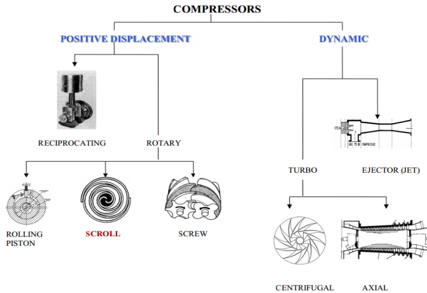
Figur 16: Kompressortyper 39
